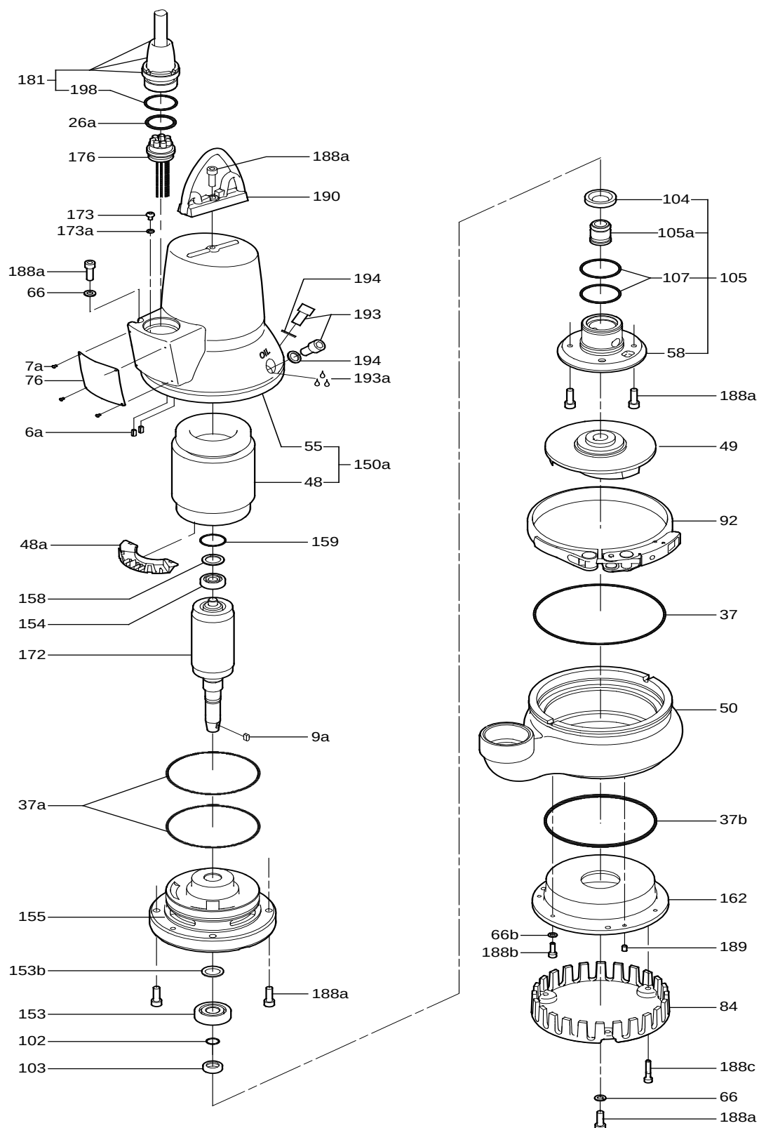
Рис. 6 Деталировка, DP10.50.09/15
