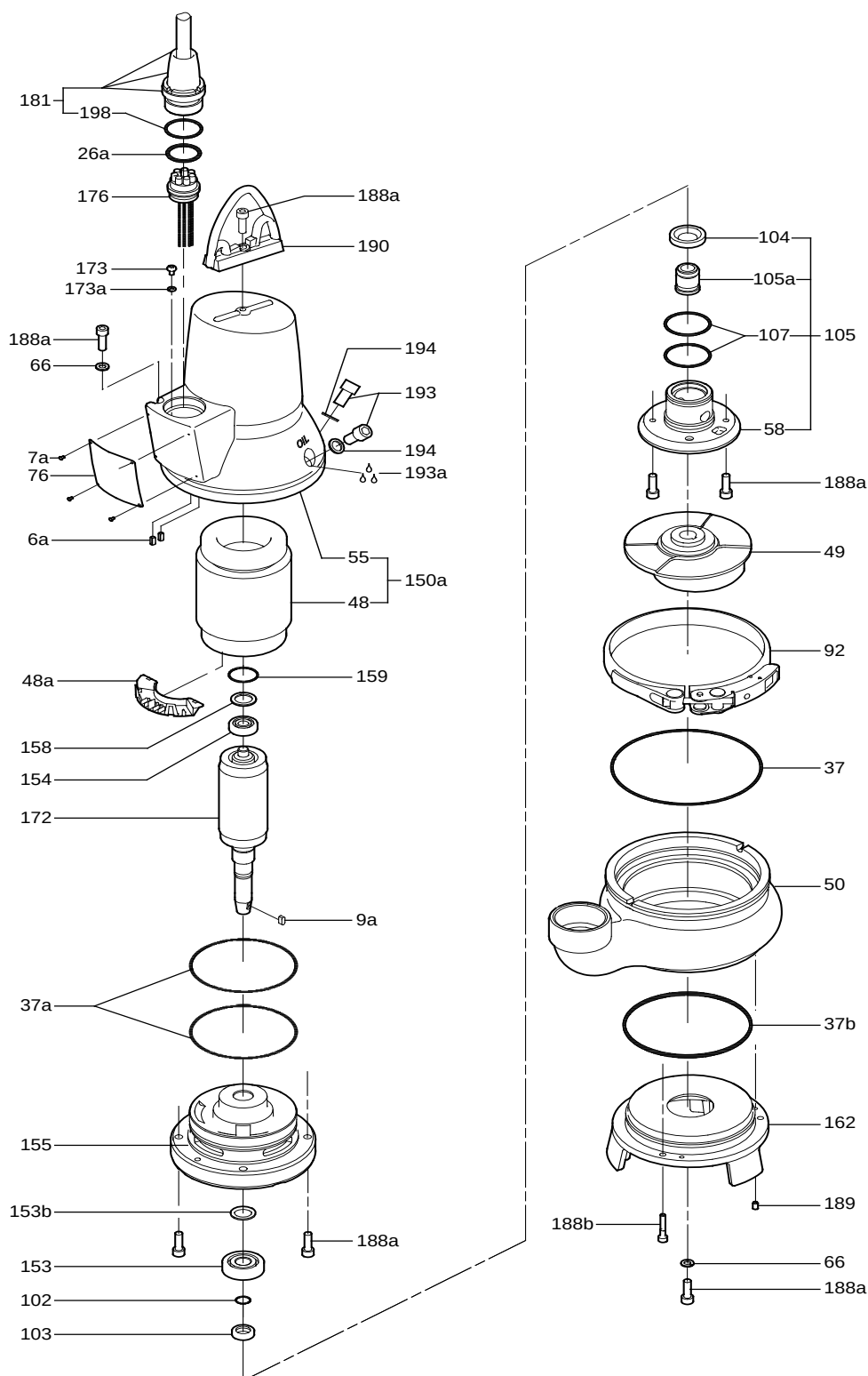
Рис. 10 Детализовка, EF
