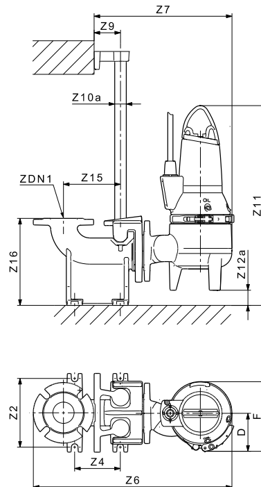
Рис. 45 Установка с одним насосом на автоматической трубной муфте
