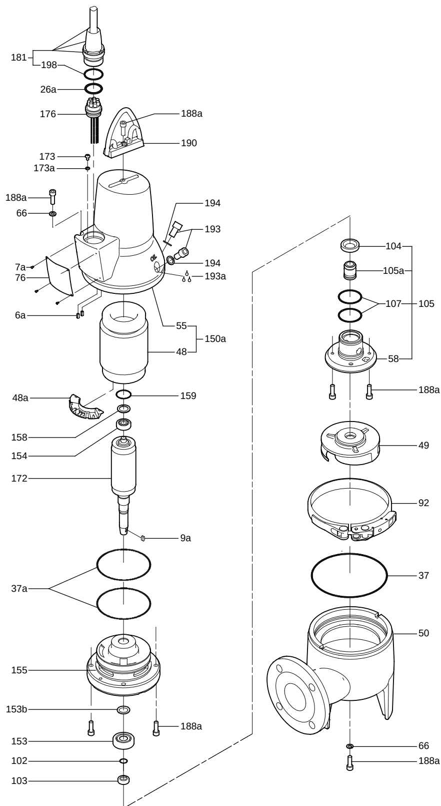
Рис. 20 Детализовка, SLV.65.65.09/11/15
