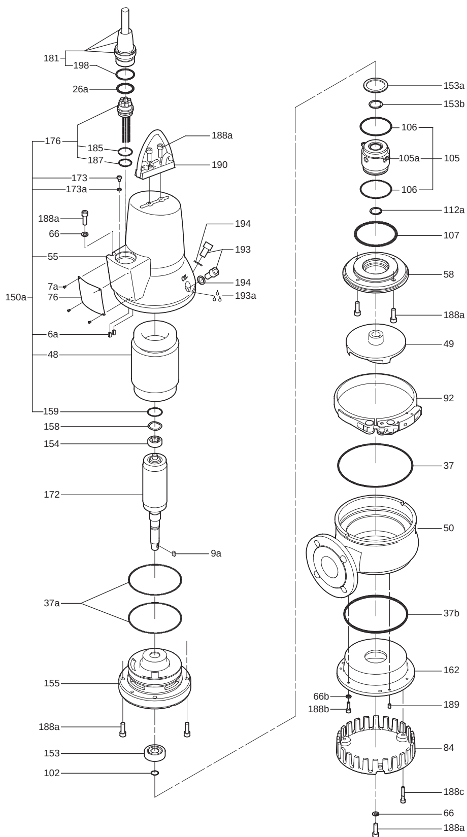
Рис. 8 Детализовка, DP10.65.26
