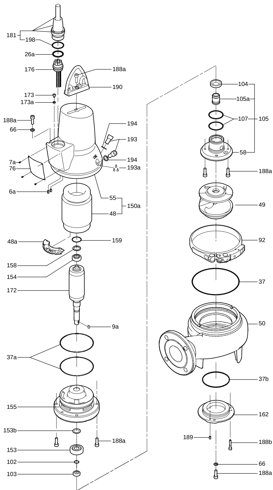
Рис. 18 Детализовка, SL1.50.65.09/11/15
