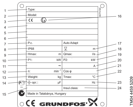
Рис. 3 Насосы DP, EF, SL1 и SLV AUTO ADAPT
