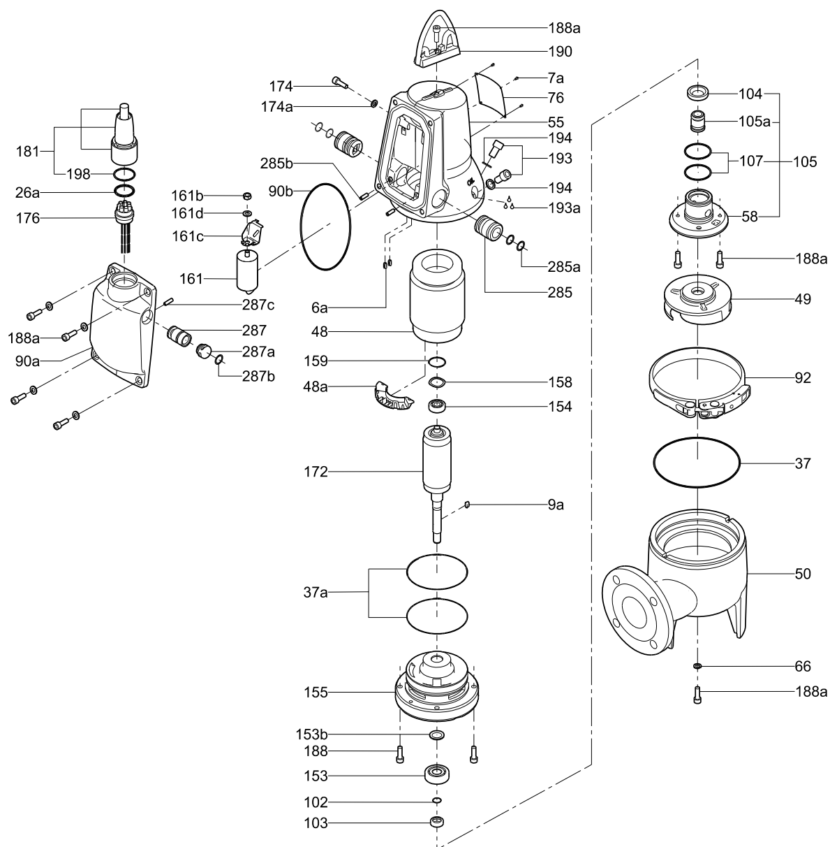
Рис. 24 Детализовка, SLV.65.65.09/11/15 AUTO ADAPT
