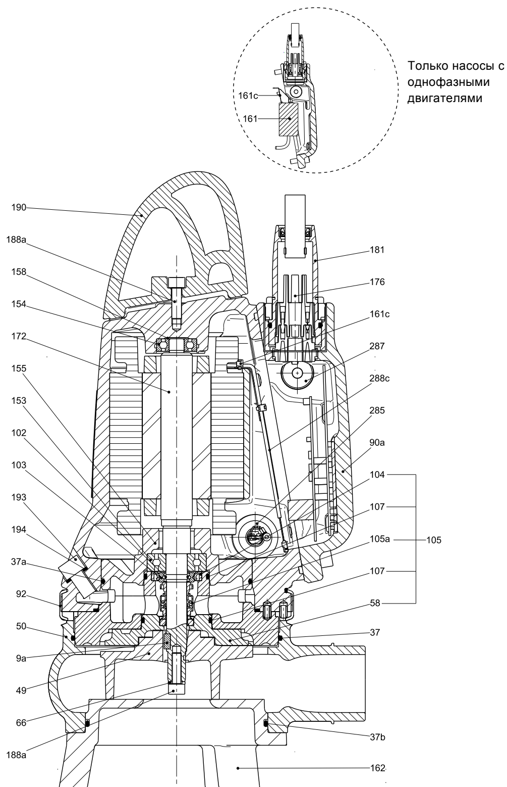
Рис. 15 Чертёж в разрезе, EF AUTO ADAPT
