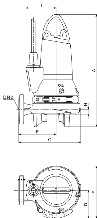
Рис. 22 Переносная установка
