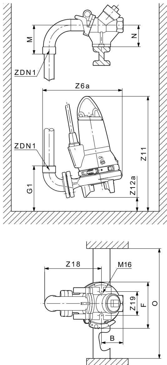
Рис. 20 Установка на надводной автоматической трубной муфте
