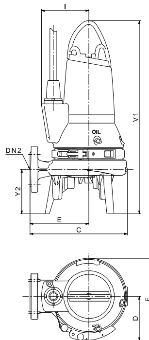
Рис. 23 Переносная установка с удлинёнными опорными ножками
