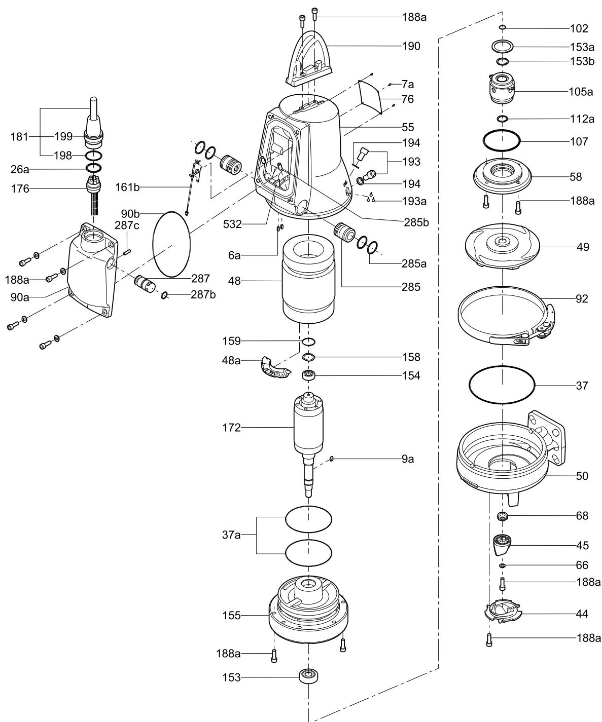
Рис. 12 Деталировка насоса AUTO ADAPT , 2,6, 3,1 и 4,0 кВт
