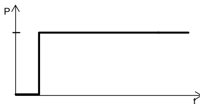
Рис. 15 Режим работы S1
