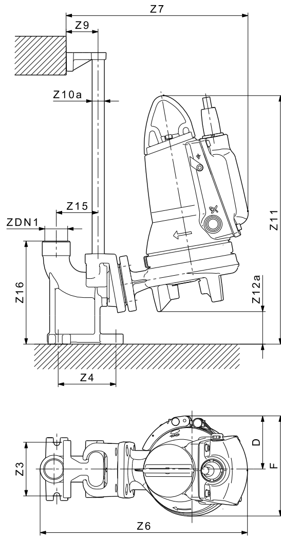
Рис. 25 Установка на автоматической трубной муфте
