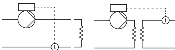
Рис. 54 "Постоянная температура"
