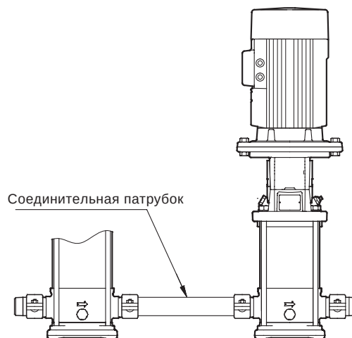
Рис. 39 Соединительный патрубок
