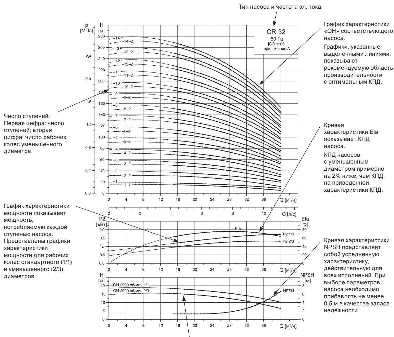
График характеристики «QH» для каждого отдельного рабочего колеса. Представлены графики для рабочих колес стандартного (1/1) и уменьшенного (2/3) диаметров.
