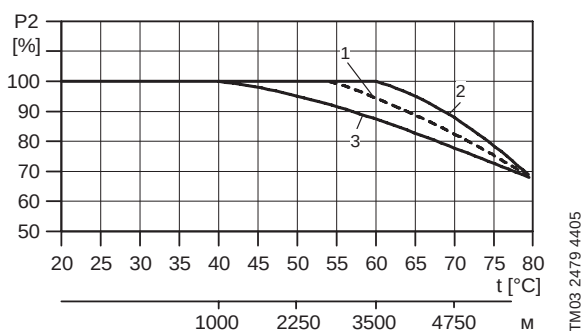
Рис. 7 Мощность двигателя P2 в зависимости от температуры/ высоты над уровнем моря
