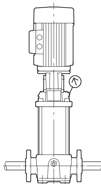
Рис. 21 Уплотнение вала
