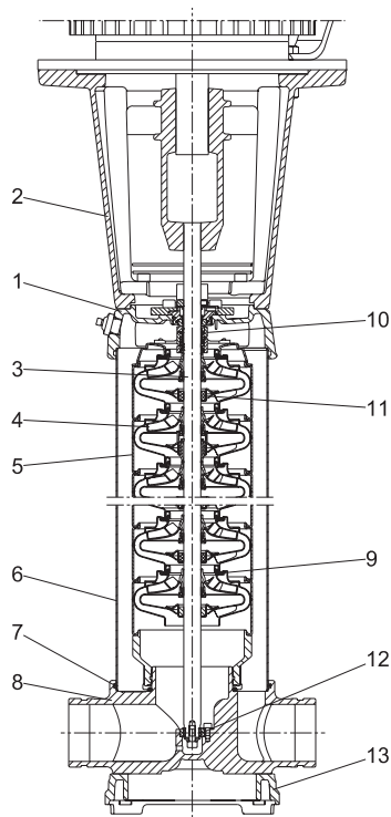
Рис. 30 Чертеж в разрезе – CRN 32, 45, 64, 90 SF
