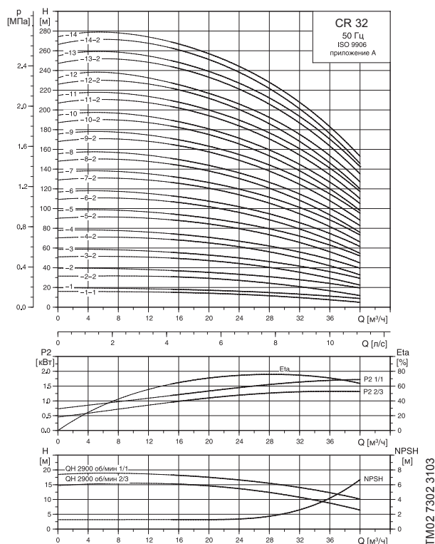
Рис. 15 Пример диаграммы характеристик
