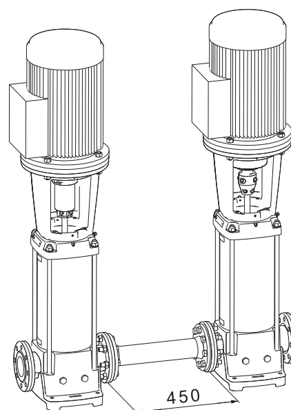
CRN питающий насос, соединительный патрубок и CRN-SF высоконапорный насос
