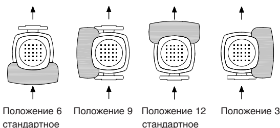
Рис. 33 Положение клеммной коробки
