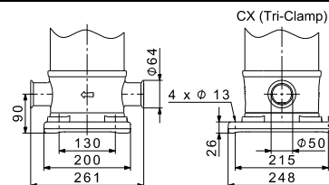
CRN питающий насос, соединительный патрубок и CRN-SF высоконапорный насос
