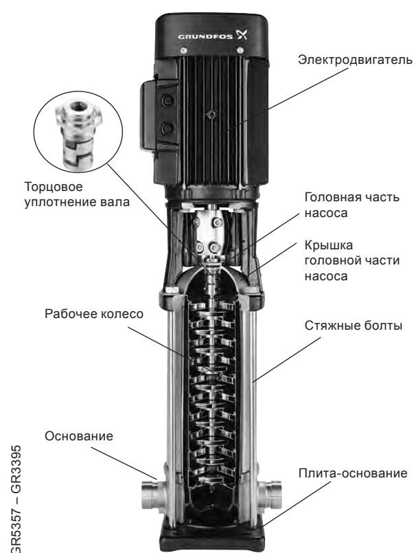
Рис. 4 Насос CR
