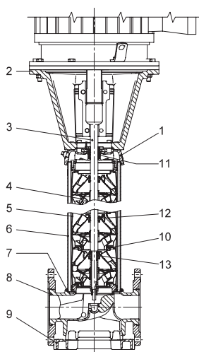
Рис. 12 Вид в разрезе
