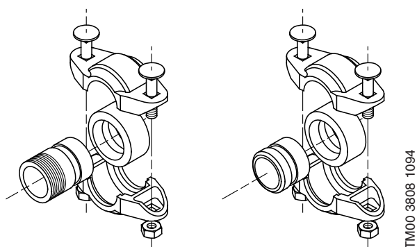
Рис. 42 Муфта PJE
