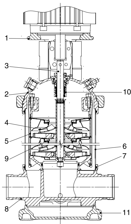
Рис. 28 Чертеж насосов CRN 3, 5, 10, 15, 20 SF в разрезе
