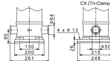
CRN-SF высоконапорный насос
