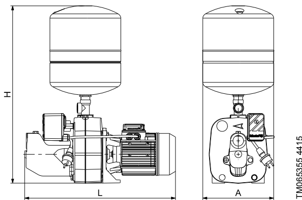
Рис. 69. JPA 5-61, 8-62 PT-V
