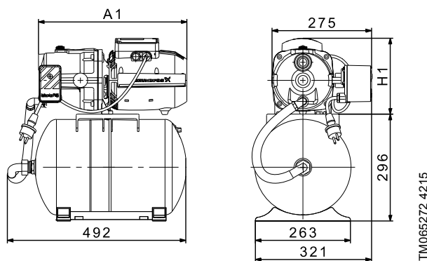
Рис. 68. JPA PT-H
