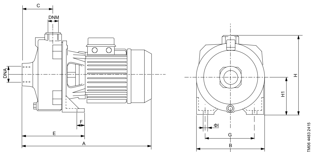
Рис. 81. NS 6-30, NS 6-40
