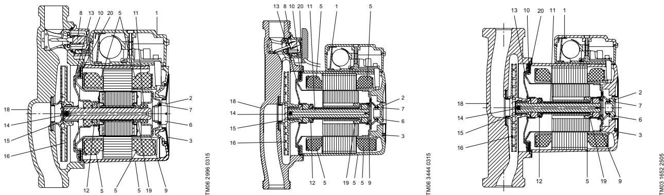
Рис. 36. Разрез насосов UPA 15-90, UPA 15-120, UPA 120
