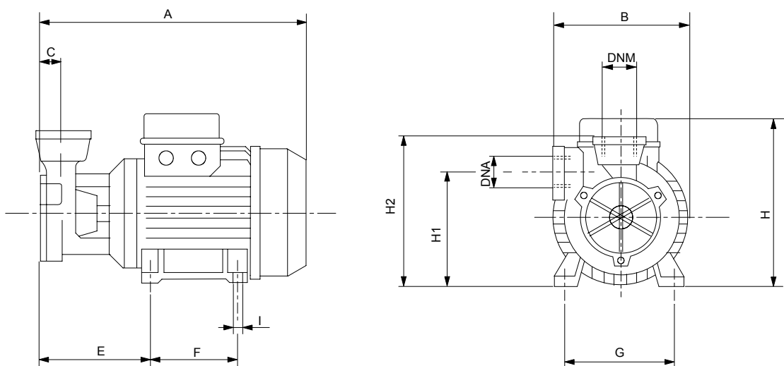
Рис. 88. PF 2-50
