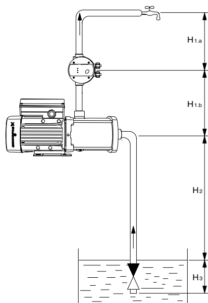
Рис. 52. Длины патрубков при монтаже установки
