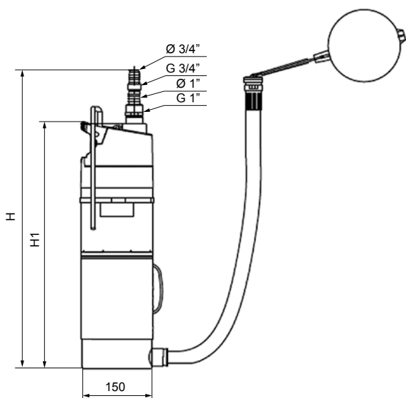
Рис. 61. Модель SBA с поплавковым сетчатым фильтром
