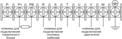
Рис. 12. Схема подключения силовой цепи трехфазного ПЧ мощностью до 15 кВт
