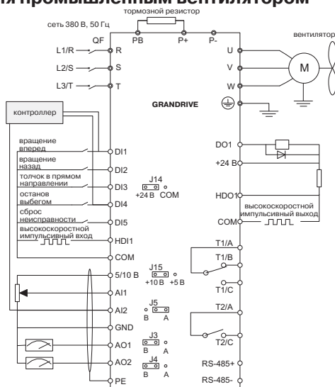
Рис. 2. Схема подключения вентилятора
