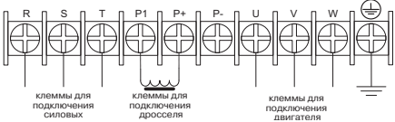
Рис.13. Схема подключения силовой цепи трехфазного ПЧ мощностью свыше 15 кВт
