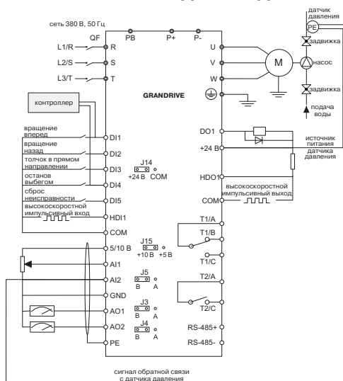
Рис. 1. Схема подключения насоса
