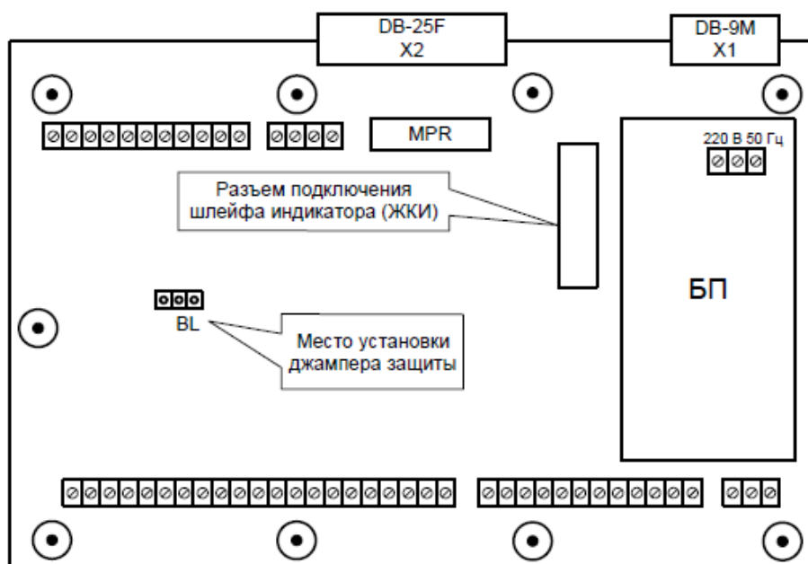
Рисунок 2. Расположение джампера в теплосчётчиках исполнения «y0xxx», где ‘у’ – буква Е,Т ‘х’ - цифра.
