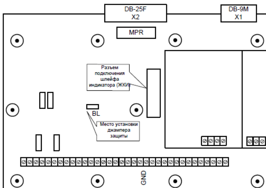
Рисунок 1. Расположение джампера в теплосчётчиках исполнения «y1xxx» и «y2xxx», где ‘у’ – буква А,Е,Т,Д, ‘х’ - цифра.
