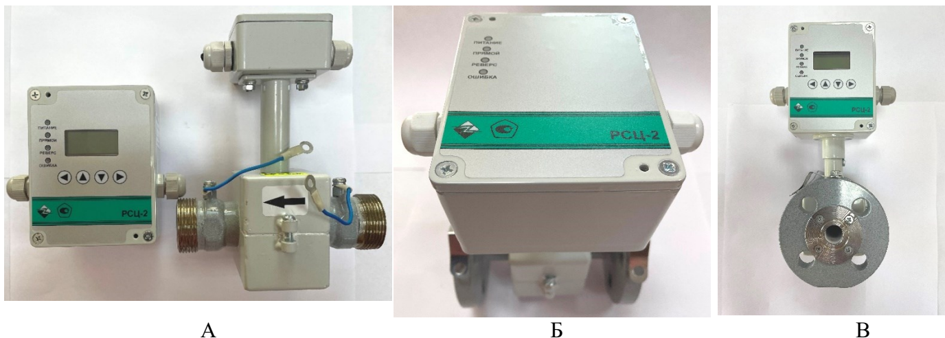
Рисунок 1 – Общий вид расходомеров: А – КС (Ф05); Б – КПГ (Ф03/Ф04); В – КПВ (Ф05)
