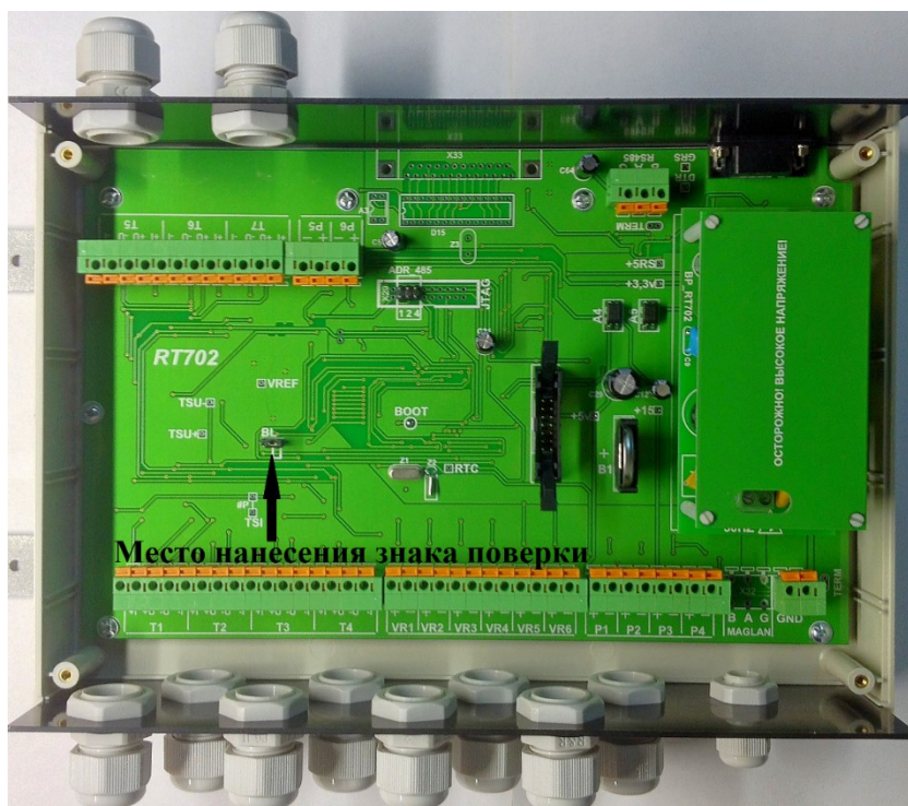
Рисунок 5 – Схема пломбировки от несанкционированного доступа, обозначение места нанесения знака поверки на переключку, расположенную на плате вычислителя без встроенного регистратора расхода
