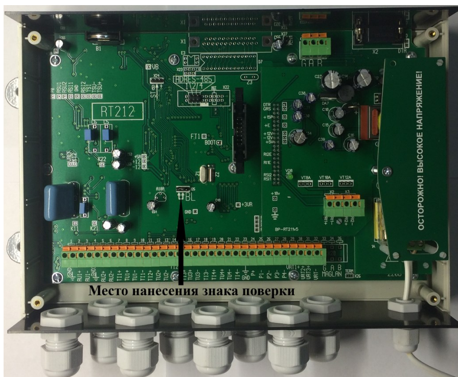
Рисунок 6 – Схема пломбировки от несанкционированного доступа, обозначение места нанесения знака поверки на переключку, расположенную на плате вычислителя с встроенным регистратором расхода
